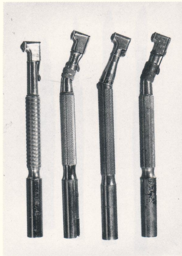
Kolenčniki, 1880 – 1960
